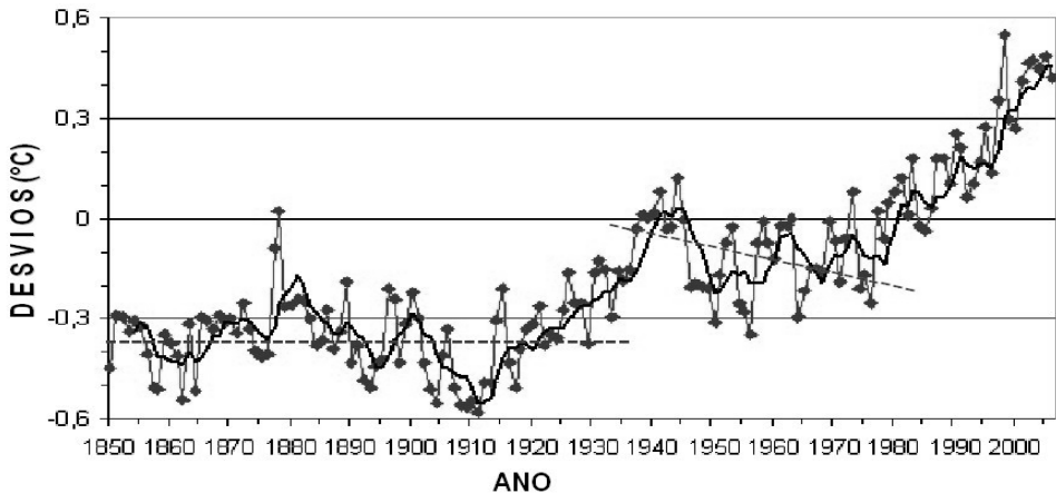
Figura 1. Desvios da temperatura média global com relação à média do período 1961-90. A curva preta é a média móvel de 5 anos e a reta tracejada (inclinada) é a linha de tendência dos desvios na fase fria da ODP, período 1947-1976 (Fonte de dados: CRU/UEA, 2007)
