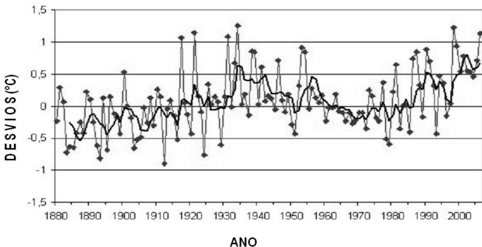
Figura 2. Anomalias de temperatura médias para os Estados Unidos (GISS/NASA, 2007)
