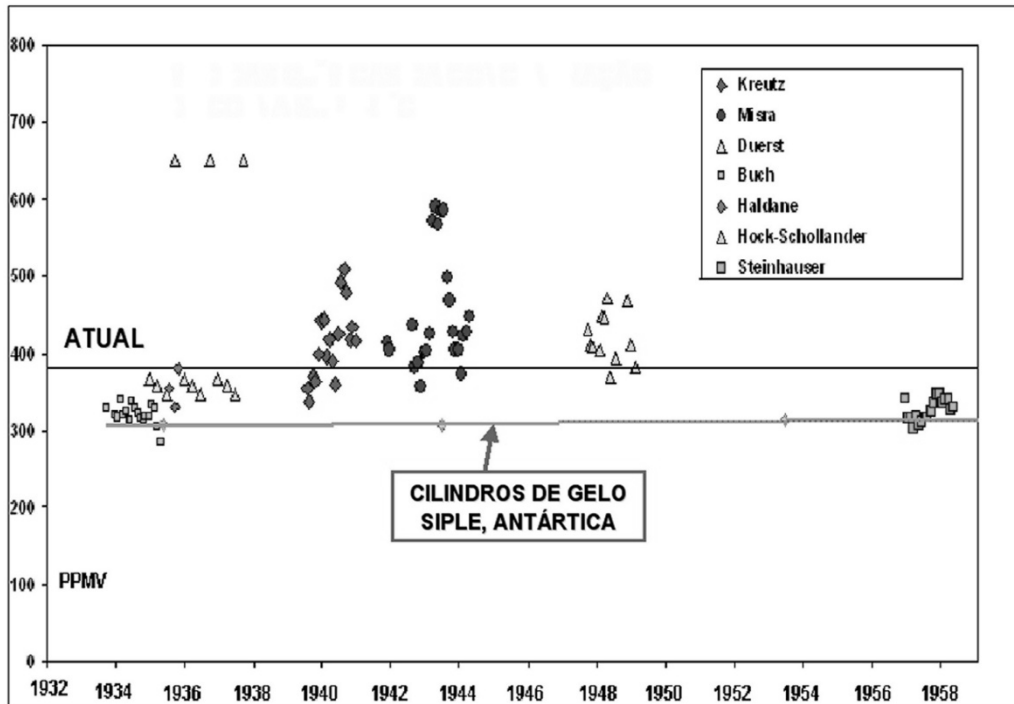
Figura 4. Medições químicas de CO 2 atmosférico, feitas por vários pesquisadores na primeira metade do Século XX, antes do início das medições em Mauna Loa, Havaí, em 1957/58.
