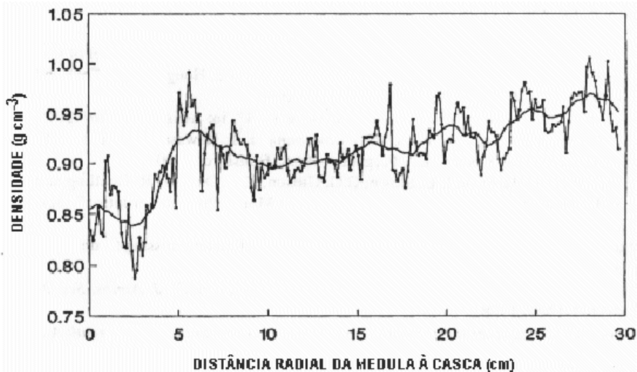
Figura 5. Variação radial da densidade da madeira dos anéis de crescimento de um jatobá-mirim , colhido em Balbina, a 170 km a noroeste de Manaus (Fonte: Ferraz et al, 1993).
